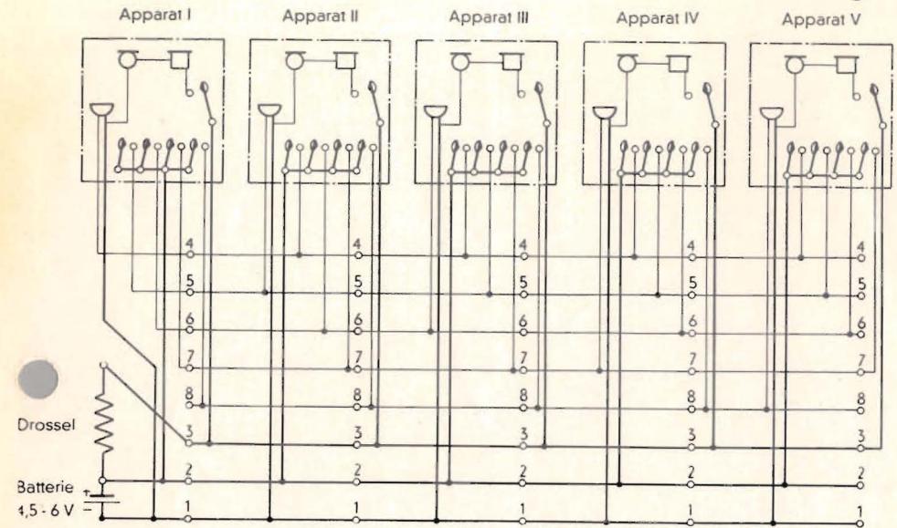
Hausteleson als Linienwähler 2 - 5 Sprechstellen
